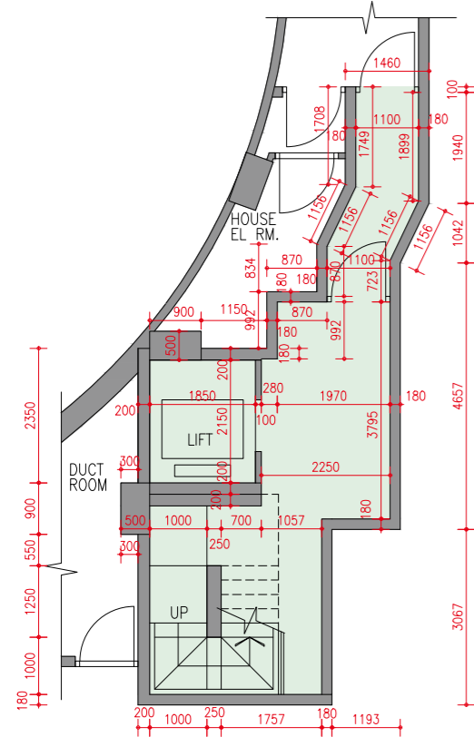
B1/F Floor Plan 地庫一樓樓面平面圖
