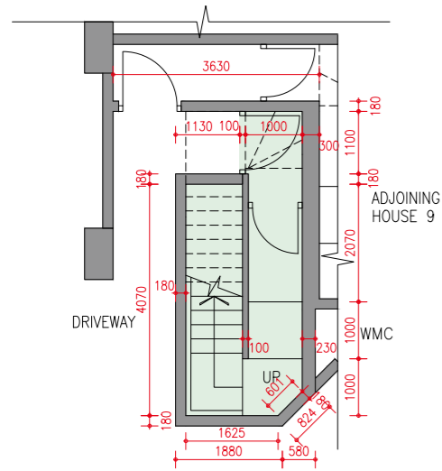
B1/F Floor Plan 地庫一樓樓面平面圖
