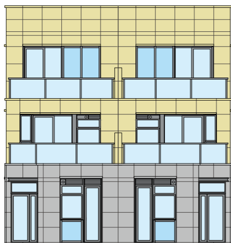
Elevation Plan 1 立面圖 1
