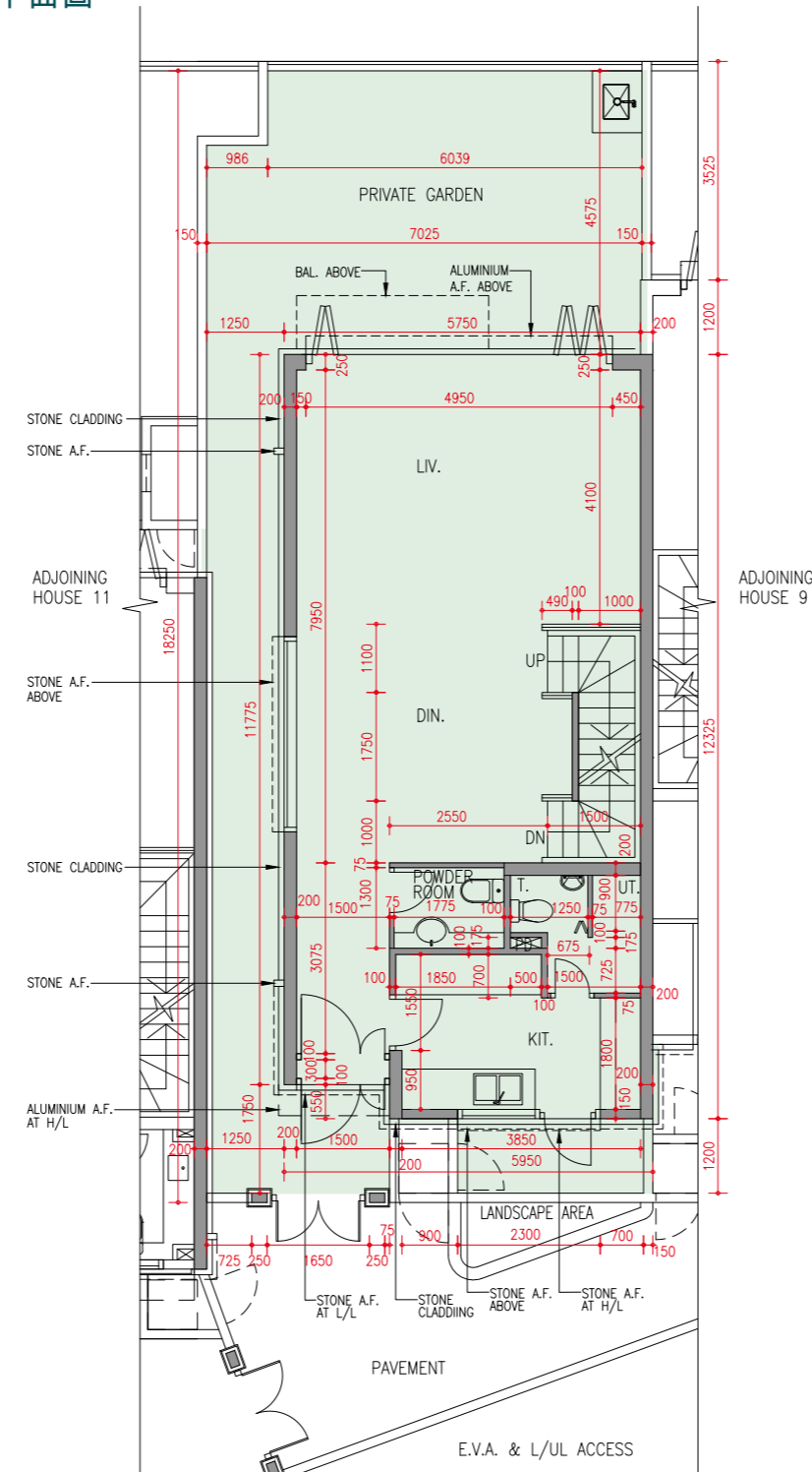
G/F Floor Plan 地下樓面平面圖
